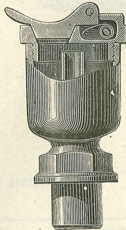
Fig. 123 Godet graisseur système ROUS
