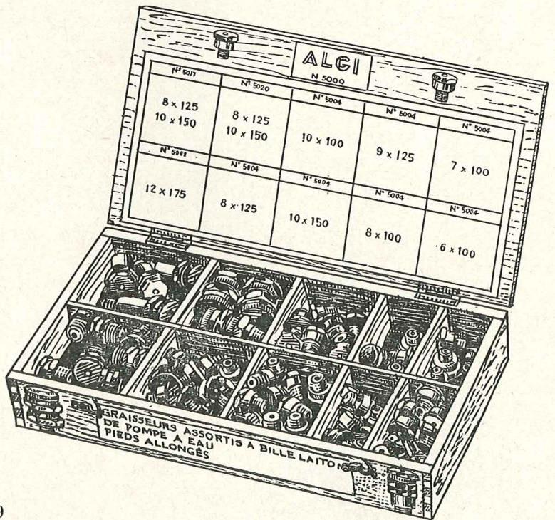
N° 5000 - Coffret bois 6x100, 7x100, 8x100, 8x125, 10x100, 10x150, 12x175 contenant 65 graisseurs à bille, 2 graisseurs de pompes à eau et 4 pieds allongés
