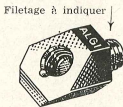
N° 5013 Equerre seule à 45° Taraudage 8 x 125
