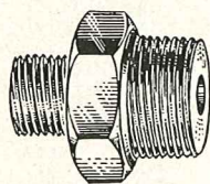
Transformateur pour agrafe 7045 N° 7153 - Deux filetages à 5/8, 18 f. et 7/16-26 f. Transformateur pour agrafe 7200 N° 7154 - Deux filetages à 5/8, 18 f. et 10/100
